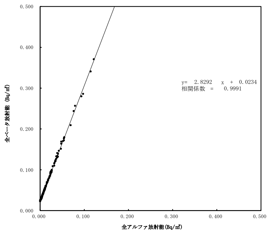
大気浮遊じんの全アルファ・全ベータ放射能の相関図 (6時間連続集じん・6時間放置後) (令和8年1月～3月) (川俣町山木屋)
