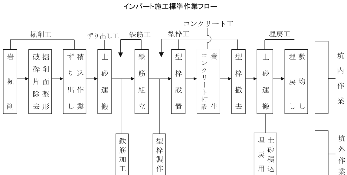
図4.2 施工フロー
