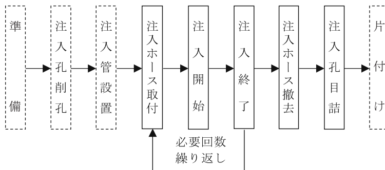
図2-2 施工フロー
