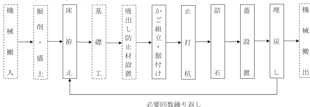
図2-1 施工フロー
