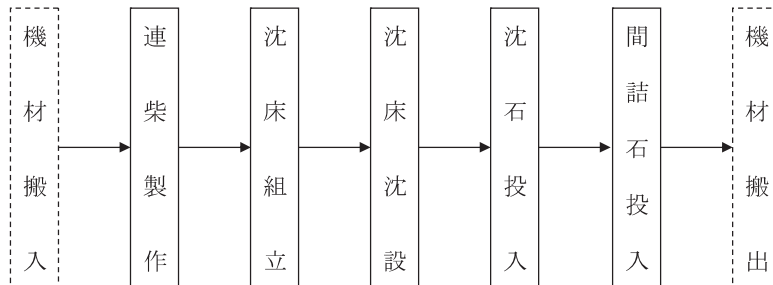
図2-1 施工フロー
