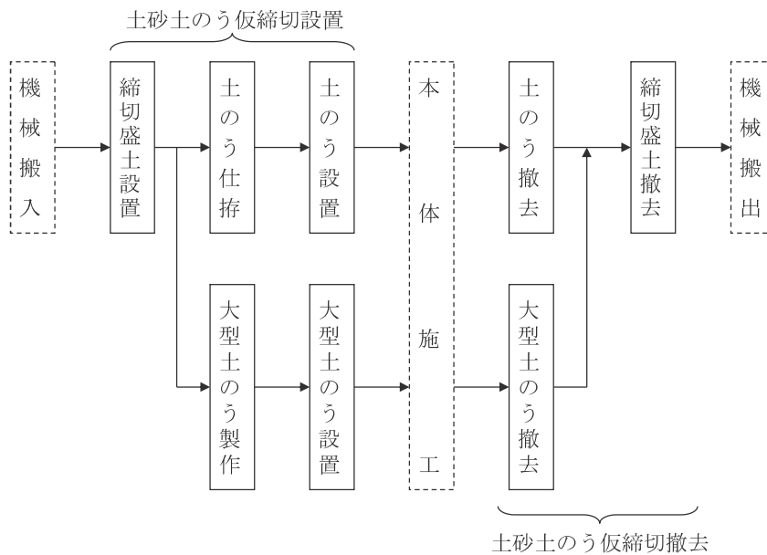
図 2-2 施工フロー
