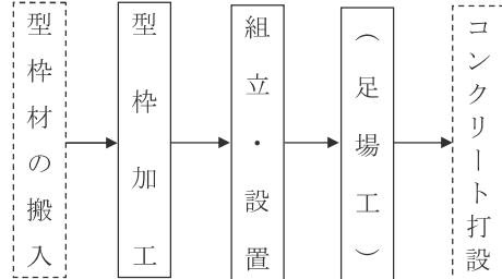
図 2-1 施工フロー
