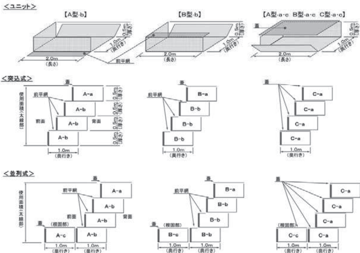
図1-1 かごマット工(多段積型)の区分(突込式・並列式), 使用面積
