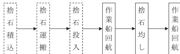
図2-1 施工フロー
