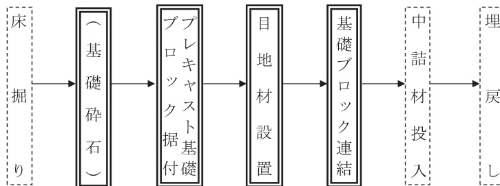
図2-2 施工フロー
