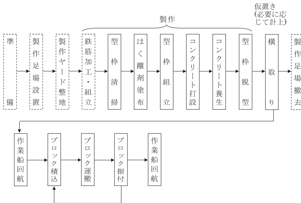
図2-2 施工フロー
