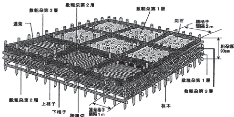
図3-1 参考図(粗梁沈床概念図)
