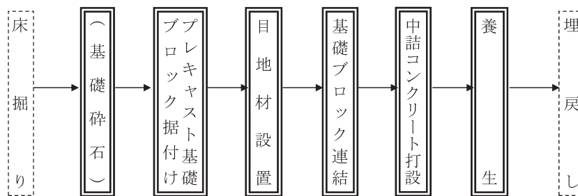
図2-1 施工フロー
