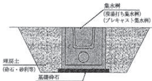
図 8-4 集水柵 構造概念図
