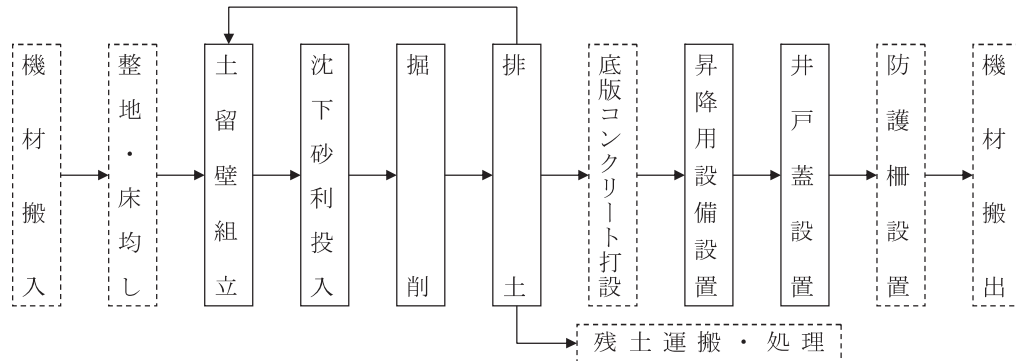
図2-1 施工フロー
