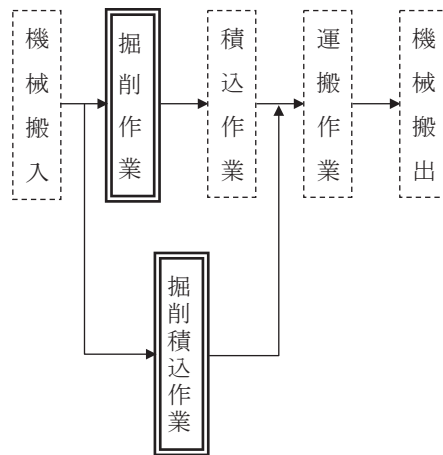
図2-1 施工フロー
