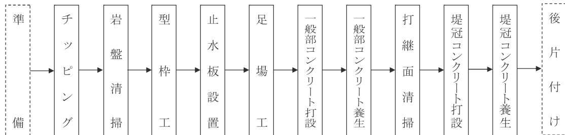
図2-1 施工フロー
