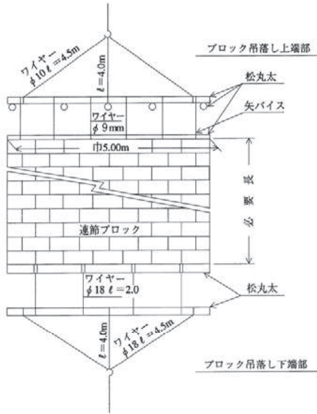
図5-1 連結ブロック水中吊落し平面図
