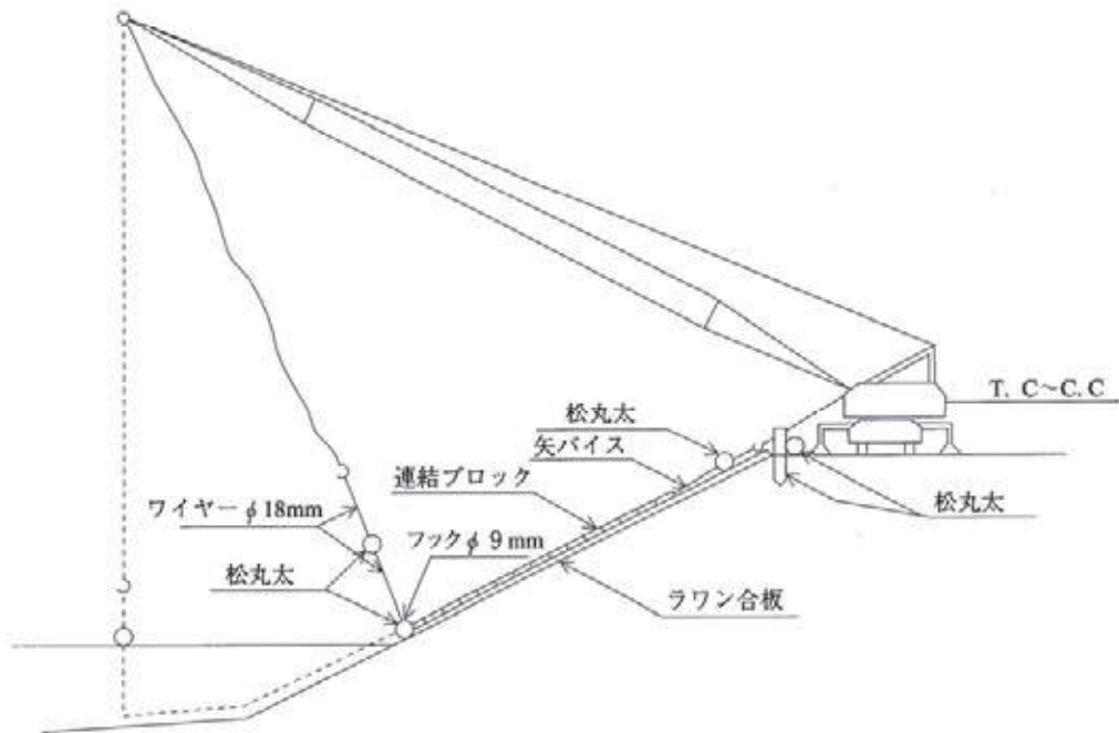
図5-2 連結ブロック水中吊落し断面図
