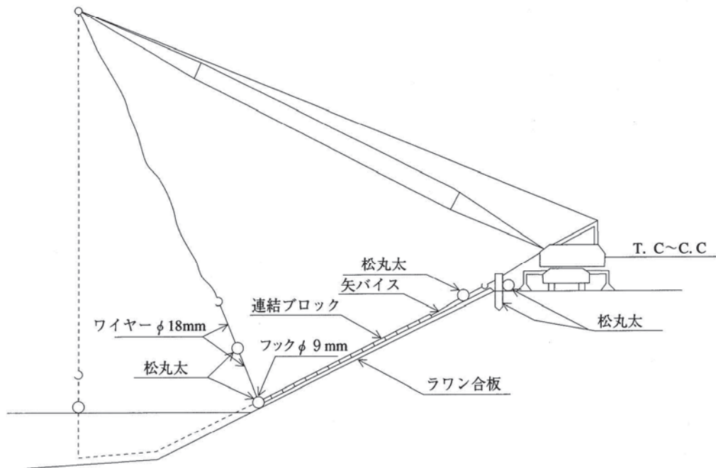
図5-2 連節ブロック水中吊落し断面図
