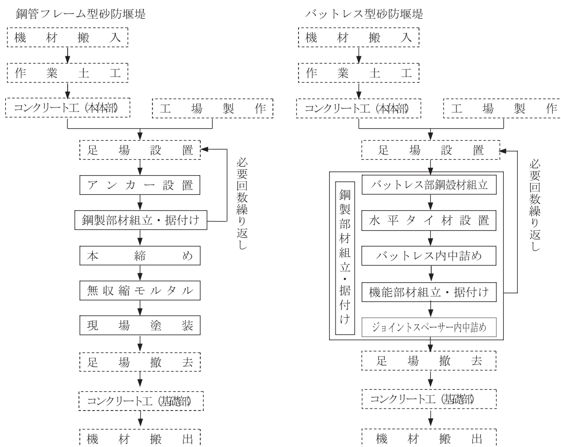
図2-1 施工フロー
