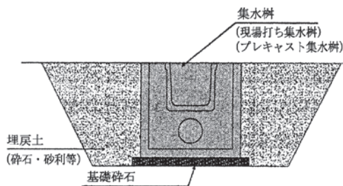
図 8-4 集水枿 構造概念図
