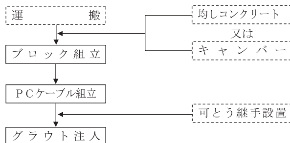
図2-1 施工フロー
