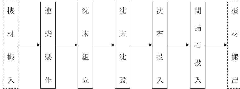
図2-1 施工フロー
