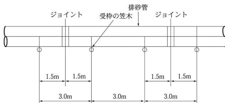
図5-1 受枠の間隔
