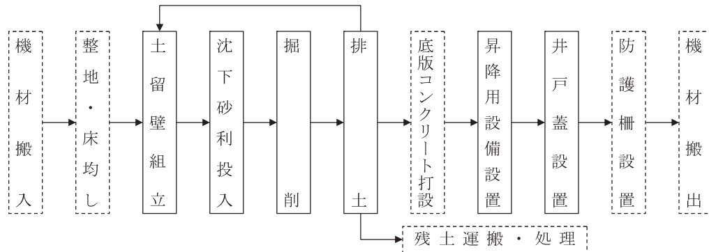
図2-1 施工フロー
