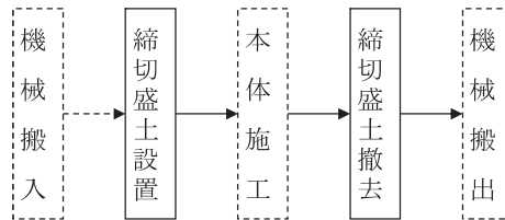
図 2-1 施工フロー
