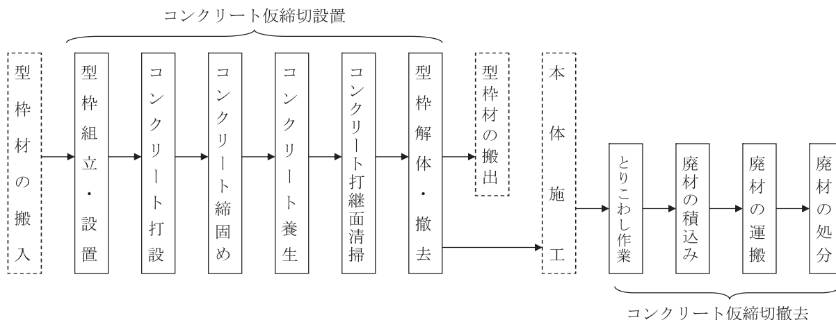
図2-1 施工フロー
