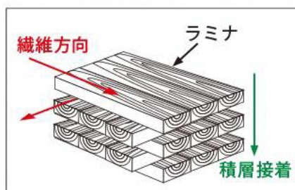
【図 7-2】 CLT の模式図
