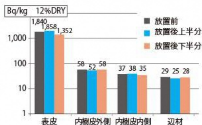
[図6-8] 林内に設置した原木のCs-137濃度変化 資料: 福島県林業研究センター林産資源部「放射線関連支援技術情報 シイタケほだ木の露地栽培に関する研究」2015年
