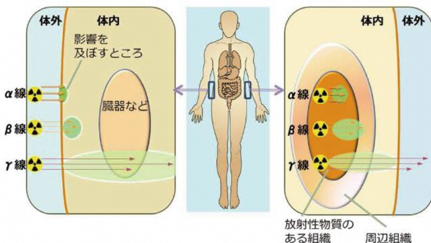
[図 2-15] 放射線の透過力と人体への影響範囲
