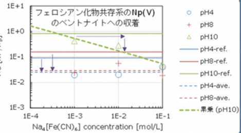
図15 人工バリアへの収着低減係数評価例
