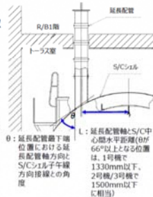
図2 S/C取水部構造の配置検討例
