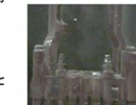
図3 4号機使用済燃料上部タイプレート締結部の外観
