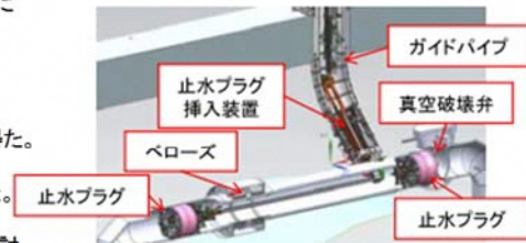
真空破壊ラインの止水プラグ施工図
