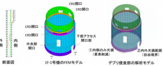
図2 RPVベDESTALの3次元FEM弾塑性解析モデル
