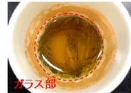
図6 ガラス化試験:ゼオライト 溶融温度約1025°C (廃棄物充填率約62wt%)
