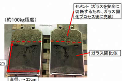
図11 パイロットスケール試験で作製されたガラス固化体
