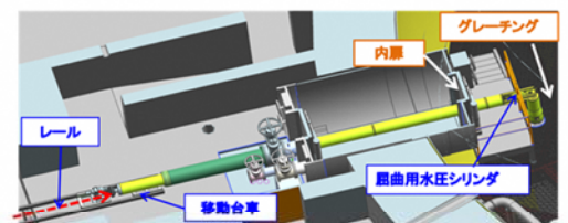
X-2ペネ内扉、グレーチング等の穿孔装置
