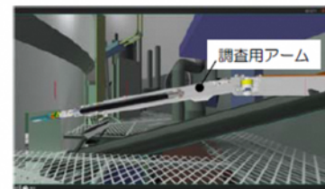
アクセス・調査装置のVRシステム
