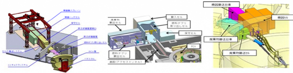
図4 燃料デブリ取り出しセルの設置イメージ
