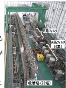
図2 実証プラント
