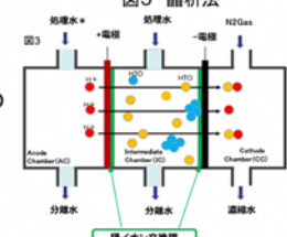
図6 電解法
