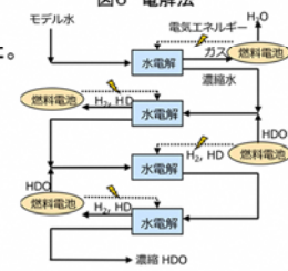
図7 燃料電池を用いた電解再結合法
