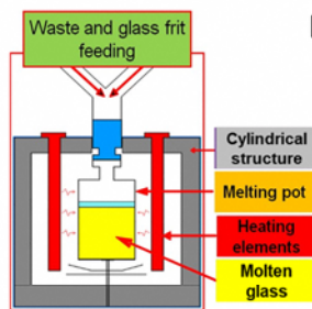
図8 In-Canガラス固化の概念図
