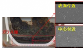
図4 ガラス化試験:鉄共沈スラリー (廃棄物充填率約35wt%)
