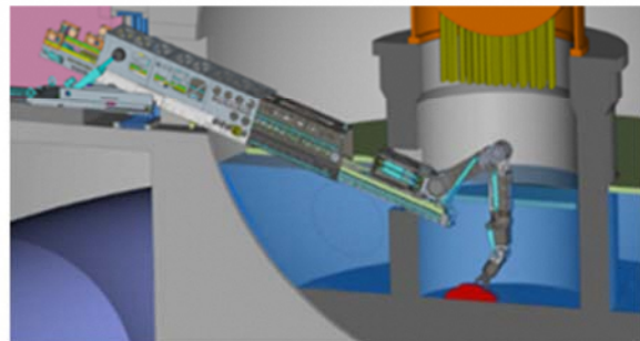
図2 気中一横アクセス工法での燃料デブリ取り出し装置の概念（検討例）
