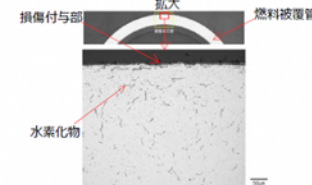
図3 水素化物析出挙動確認試験結果の例 (照射試験片, 300℃, 冷却速度0.04℃/h, 周方向応力70MPa, 損傷付与, 海水付着, 互摩因着)
