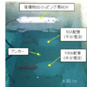
水中遊泳型調査装置と計測装置との組合せ試験例
