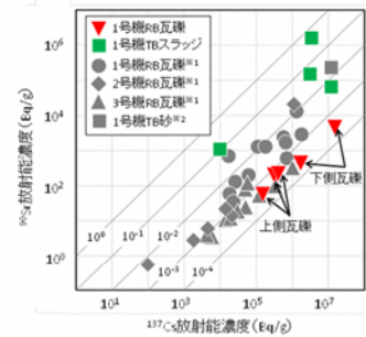
図20 瓦礫中の 90 Sr/ 137 Csと放射能濃度比
